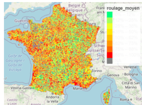
FIGURE 4.9 – Cartographie de la fréquence de conduite
