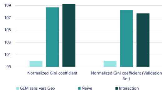
FIGURE 4.22 – Comparaison des indices de Gini normalisés (base 100 avec pour référence les valeurs des indicateurs du modèle initial sans variables géographiques)
