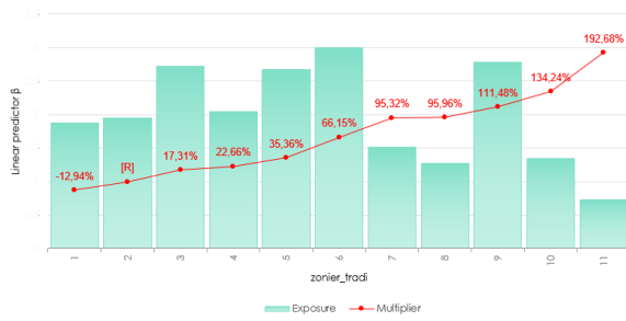
FIGURE 5.23 – Courbe des facteurs multiplicatifs des modalités du zonier traditionnel
