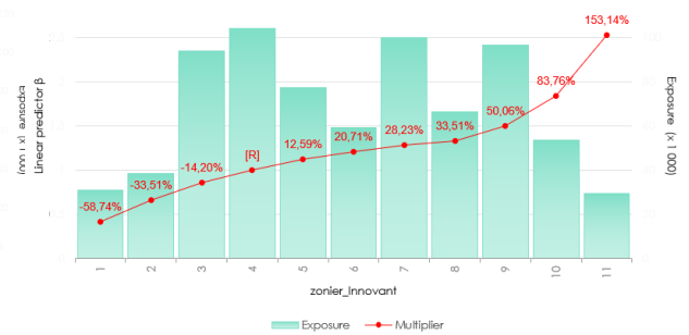
FIGURE 5.24 – Courbe des facteurs multiplicatifs des modalités du zonier innovant
