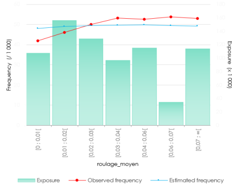
FIGURE 4.8 – Analyse des valeurs observées et estimées de la fréquence de sinistres sur la Fréquence de conduite
