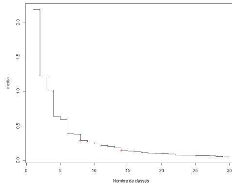
FIGURE 5.12 – Perte d’inertie inter-groupe en fonction du nombre de zones
